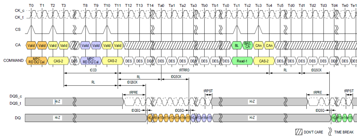
Figure 109. DQ Read Training Timing: Read DQ Cal. to Read DQ Cal. / Read
